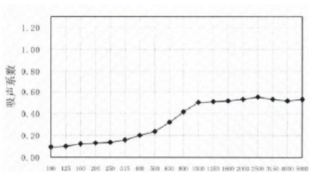
▲ 天然软木常规板
